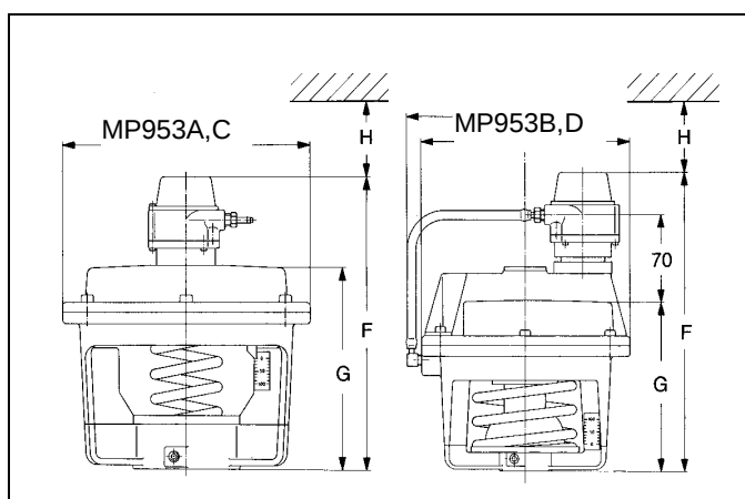
Рис. 2 MP953A,C/MP953B,D
