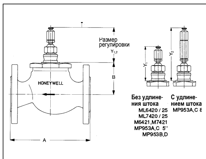
Рис. 1 V5328A
