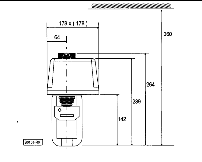
Рис. 4 M6421A/M7421A
